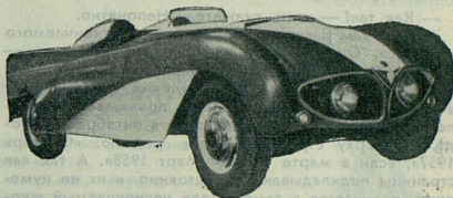
Съемный кузов спортивного автомобиля «ЗИЛ-11», сделанный из полиэфирного стеклопласта.
